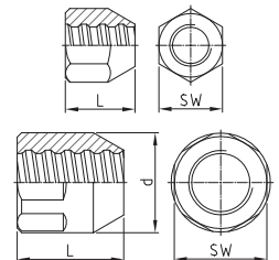
Anschweißstück SW welding bolt hexagonal
