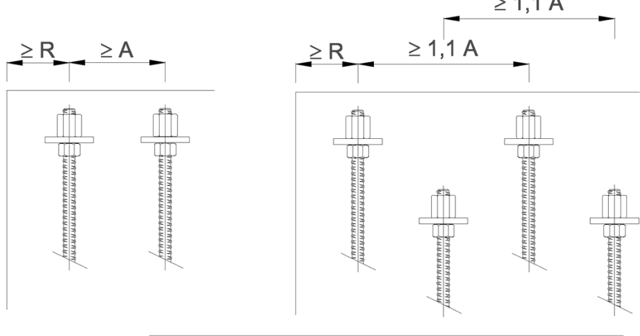
versetzte Verankerung
