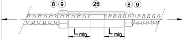
Bild 5 Muffenstoß - Spannschloß Ø12 - 50
