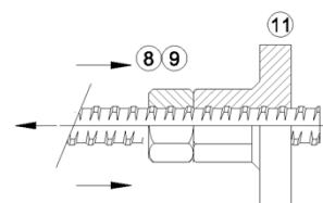
Bild 3 Ø12 - 50
