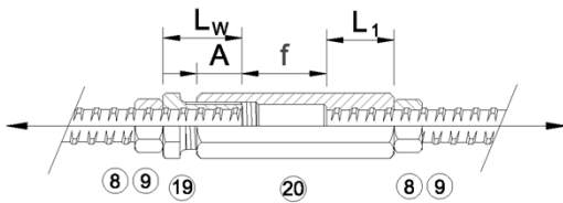
Bild 5 Muffenstoß - Spannschloß Ø12 - 50
