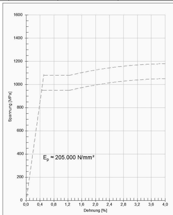
Bild 2: Prinzipieller Spannungs-Dehnungsverlauf
