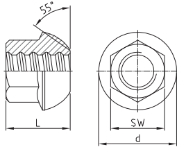
Kugelbundmutter 55° domed nut 55°
