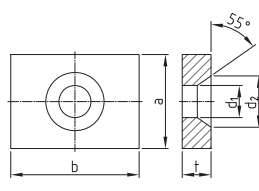
Ankerplatte rechteckig 55° anchor plate rectangular 55°
