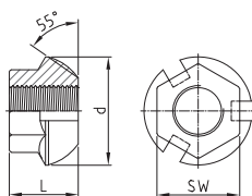
Kugelbundmutter 55° mit Verpressnuten domed nut 55° with grout slots
