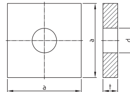
Ankerplatte gerade anchor plate flat
