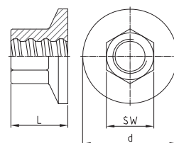
Ankerstück anchor piece
