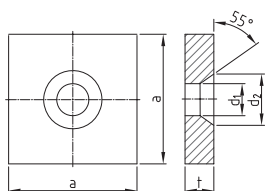
Ankerplatte quadratisch 55° anchor plate square 55°
