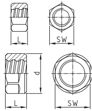
Haltemutter fix nut
