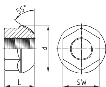
Kugelbundmutter 55° dome nut 55°
