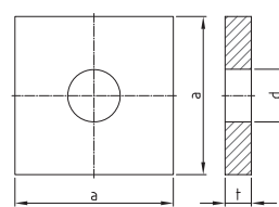
Ankerplatte gerade anchor plate flat
