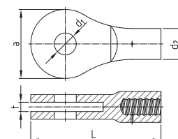
Gabelstück fork piece
